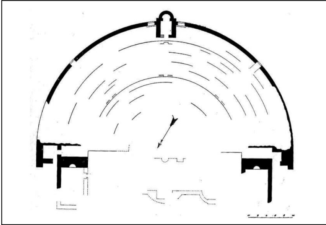
الشكل رقم (07): المخطط العام لمسرح روسيكاد
