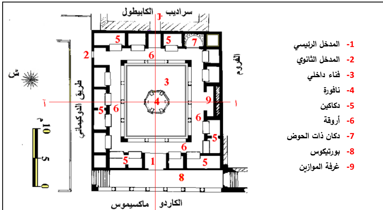
الشكل رقم (04): مخطط عام لسوق الإخوة كوزينيوس بمدينة كويكول
