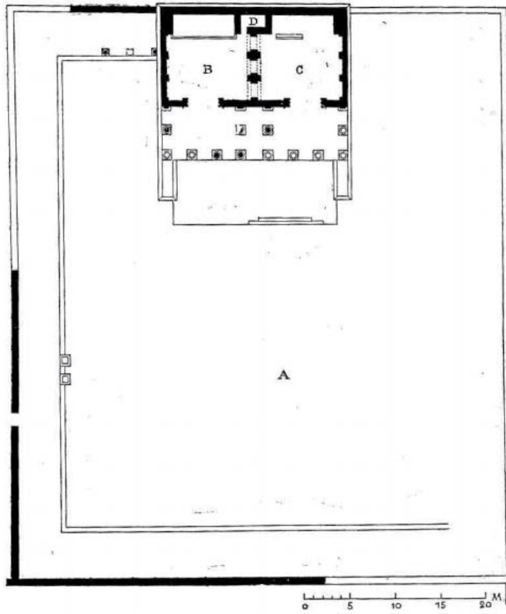
الشكل رقم (02): مخطط عام لمعبد الكابتول بلمبايزيس عن: GSELL (St.), M.A.A., Op-cit, P. 144
