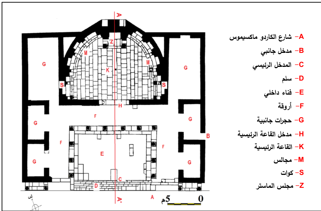
الشكل رقم (09): مخطط عام لمكتبة مدينة تاموقادي.
